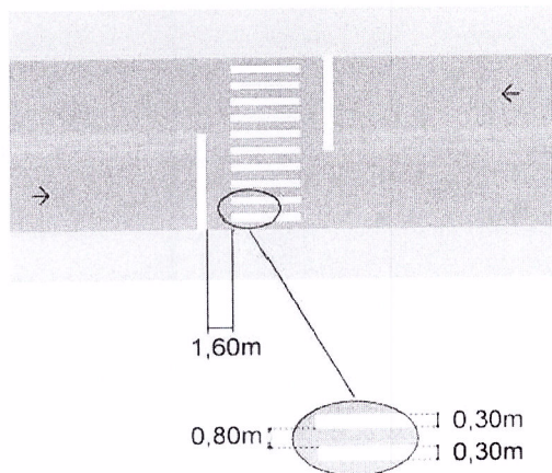
Faixa de travessia de pedestres (FTP)
