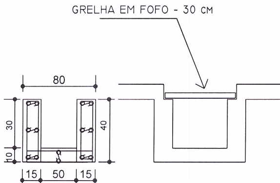
DETALHE FERRAGEM PONTO DE DRENAGEM ESCALA S.N
