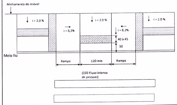
RAMPA NO PASSEIO ≤ 2,20 m
