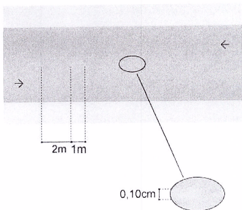
Linha simples seccionada (LFO-2)
