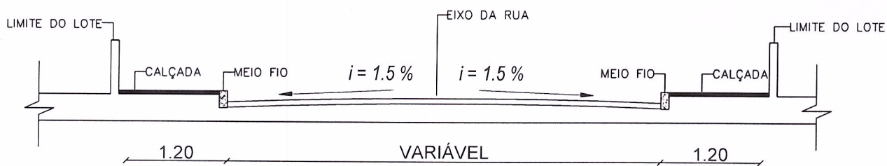
DET. TIP. VISTA LONGITUDINAL
