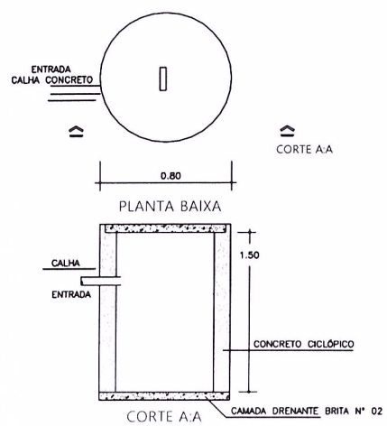
DETALHE BUEIRO PONTO DE DRENAGEM ESCALA S.N
