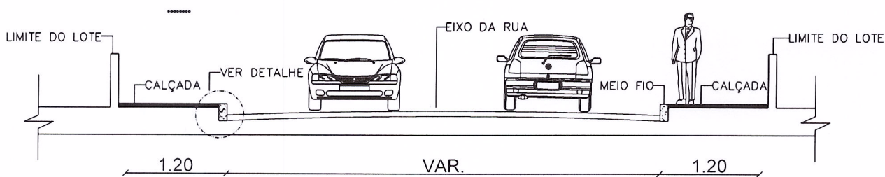
DET. TIP. VISTA LONGITUDINAL
