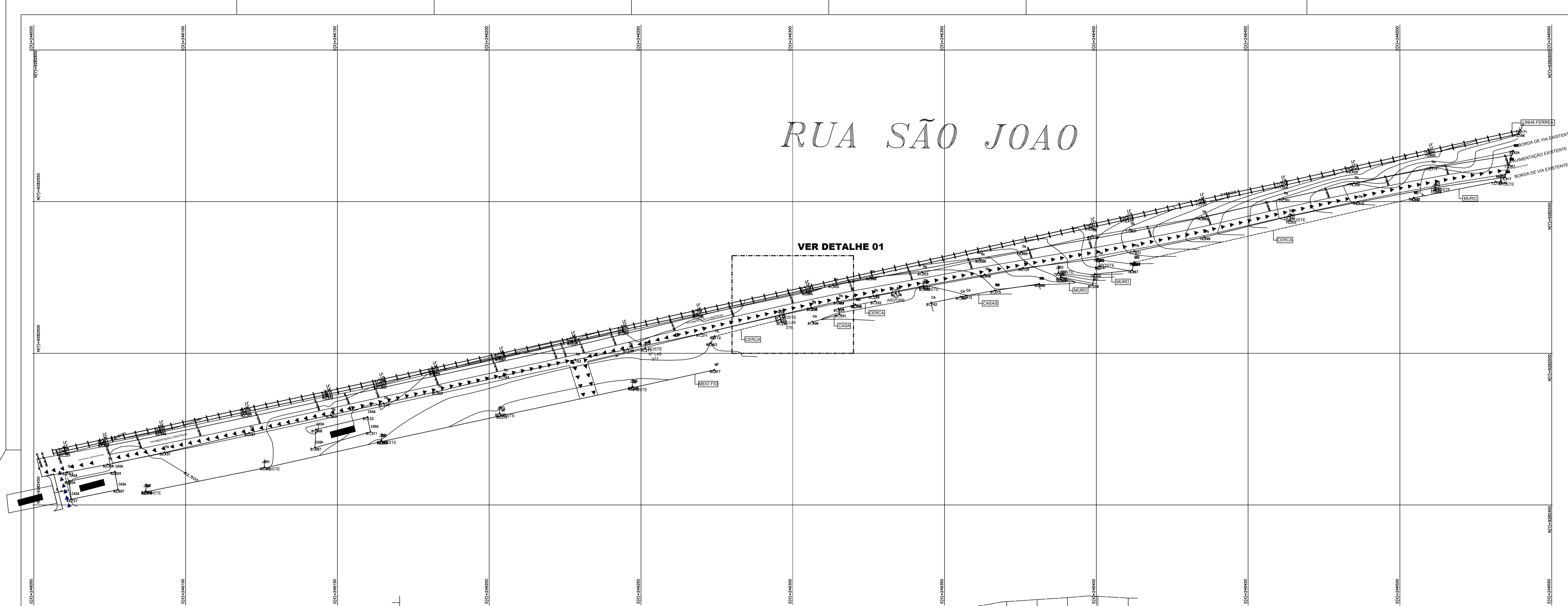
PROJETO DE PAVIMENTAÇÃO ESCALA ..... 1:500
